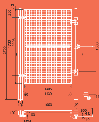
PORTONES PEATONALES h223
