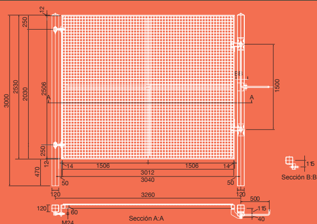
PORTONES DE ENTRADA DE VEHÍCULOS h253
