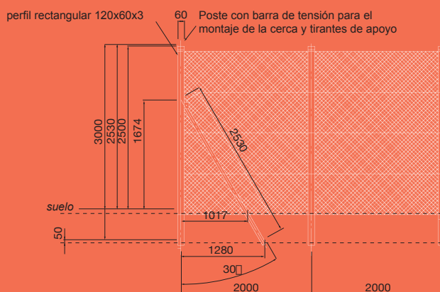
Separadores perimetrales externos h 2500 mm
